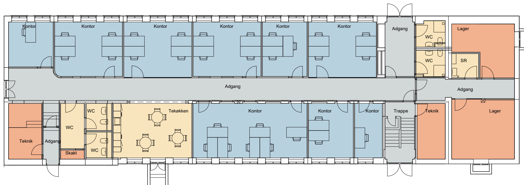
Stueplan
